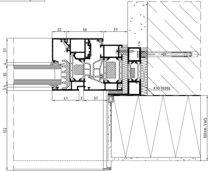
Ansicht M1:10
