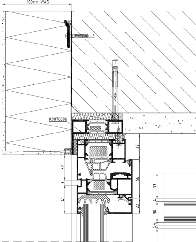
Vertikalschnitt A - B
