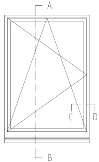
Ansicht M1:10
